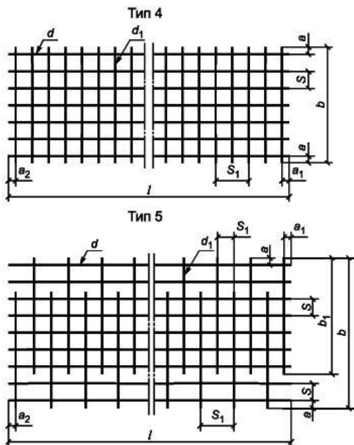
Рисунок 2* - Легкие сетки
