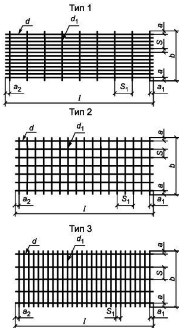
Рисунок 1* - Тяжелые сетки
